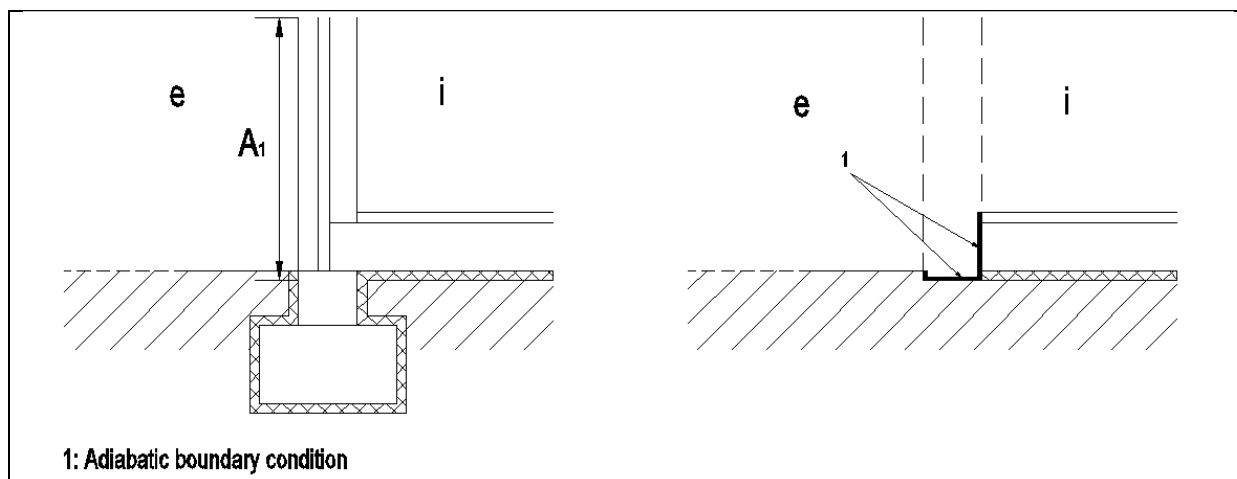
Figuur 0.2 Aanpassing van het werkelijke detail ter berekening van de U-waarde van de vloer op volle grond.
