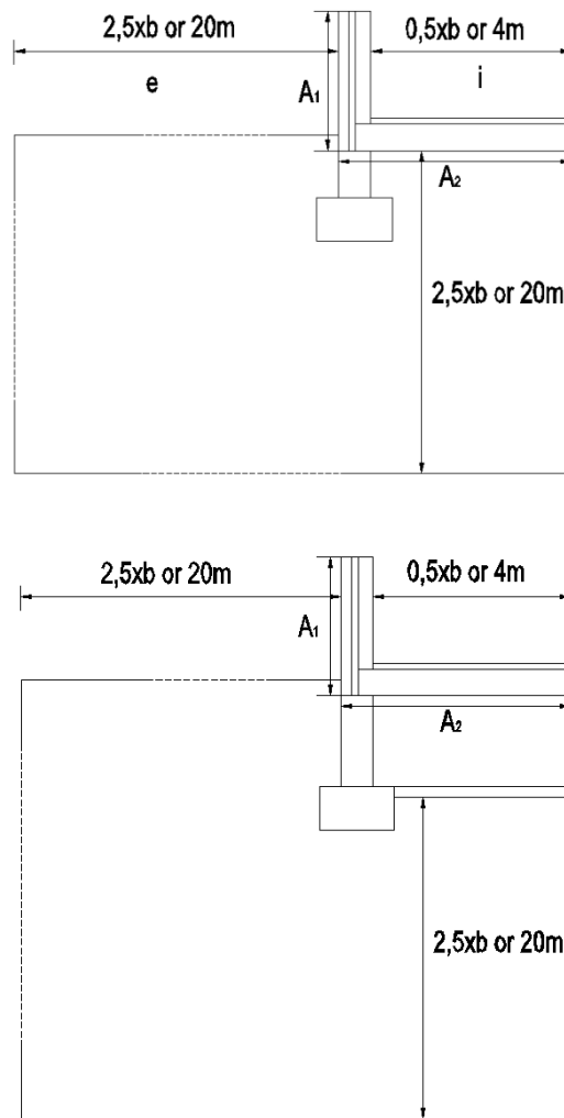
Figuur 0.3 Positie van de snijvlakken van een geometrisch model waarin het grondmassief betrokken is (boven: vloer op volle grond – onder: vloer boven kelder).
