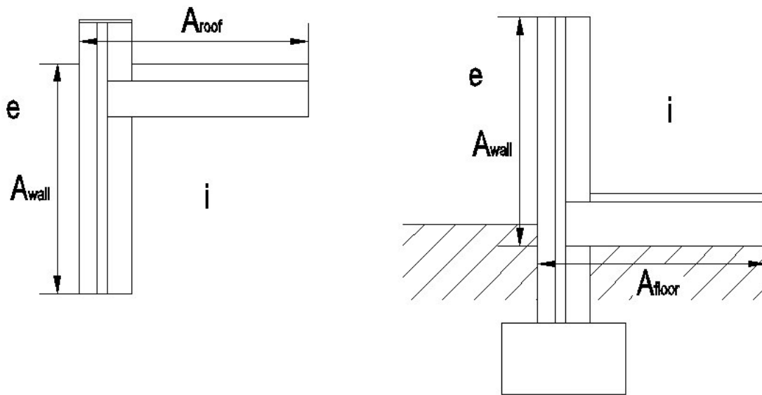
Figuur 0.1: Voorbeeld buitenafmetingen bij aansluiting plat dak met gevel (links) en bij de funderingsaanzet van een vloer op volle grond (rechts).
