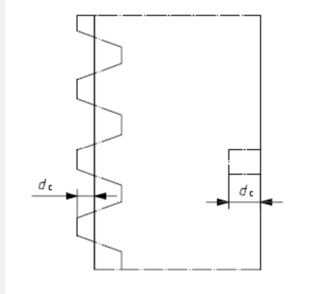
Figuur 0.4 Het uitvlakken van geprofileerde oppervlaktes (links) of een lokale dikteverandering (rechts) aan het binnen- of buitenoppervlak (Figuur: NBN EN ISO 10211:2008) .
