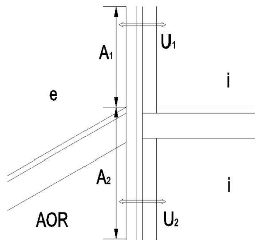
Figuur 0.1 Aanduiding van de gebruikte termen in het geval een aangrenzende onverwarmde ruimte.
