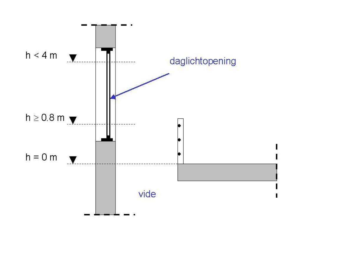
Figuur 1 Projectie van de bovenkant van de vloer op de gevel (bv. bij vides) en begrenzing van de te beschouwen minimale en maximale hoogte van de (equivalente) verticale daglichtopening
