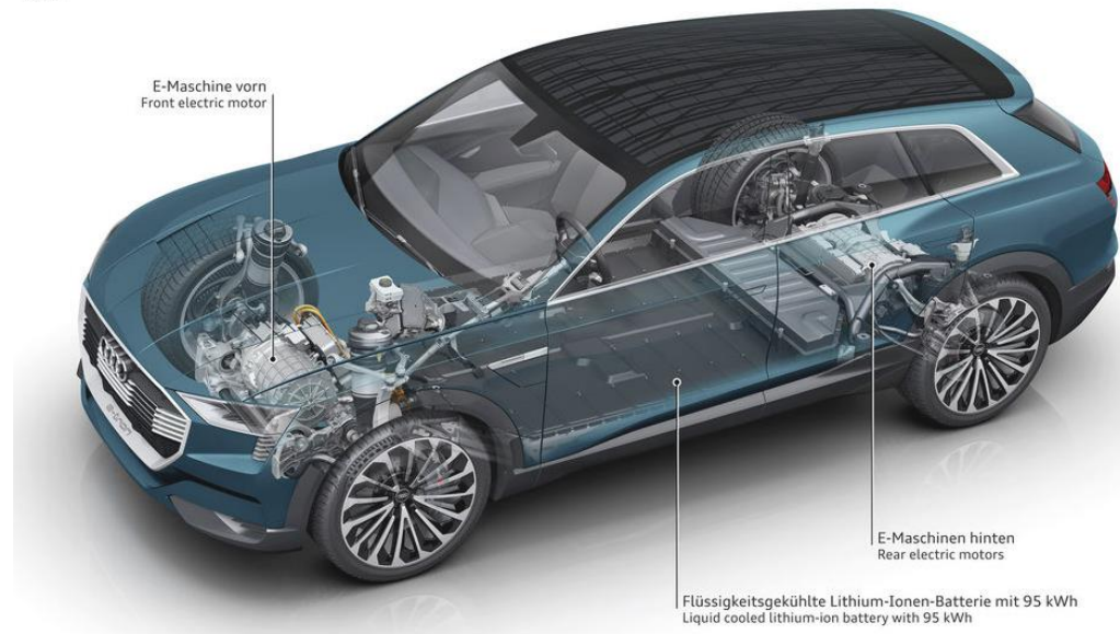
Audi e-tron quattro concept elektrischer Antriebsstrang mit bis zu 370 kW Leistung Electric drivetrain with up to 370 kW 09/15
