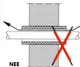
Doorvoerkoker met te grote diameter t.o.v. die van de leiding
