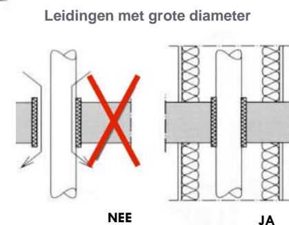
Doorvoerkoker kleiner dan de dikte van de wand
