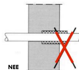
Doorvoerkoker kleiner dan de dikte van de wand
