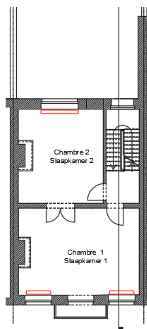
Niveau +1
