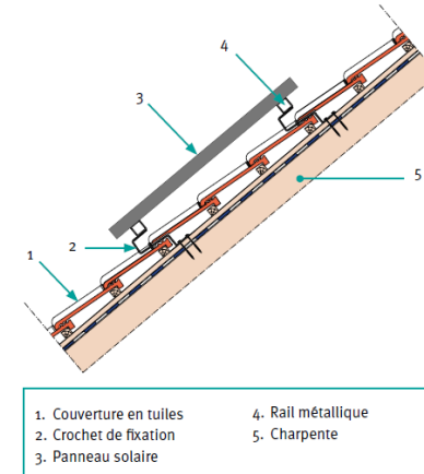
Fig. 2 Montage en surimposition.
