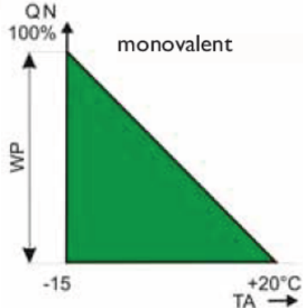
Système de distribution de la chaleur t_v < 60\text{ °C}
