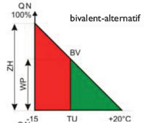
Système de distribution de la chaleur t_v > 60\text{ °C}
