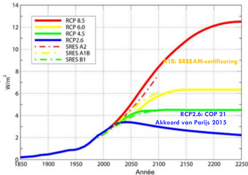
Afbeelding 3: Na 2006 komen de ononderbroken lijnen overeen met de zogenaamde RCP-scenario's (Representative Concentration Pathways) en de stippellijnen met de SRES-scenario's - bron:
