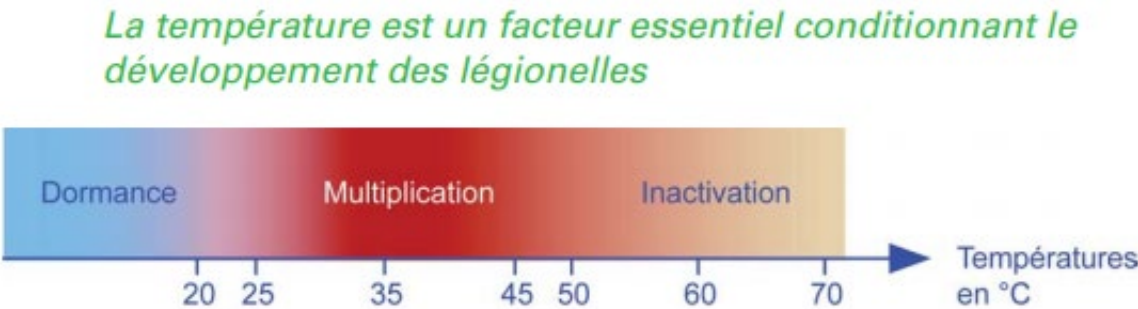
▲ Figure 13 : La croissance des légionelles en fonction de la température. L’optimum de croissance se situe entre 25 et 45°C environ.
