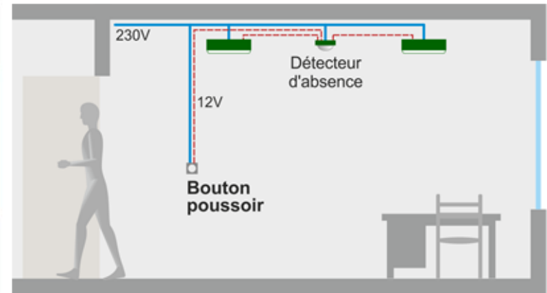
Voorbeeld van semi-automatisch beheer van de in- en uitschakeling van de verlichting in langdurig bezette lokalen
