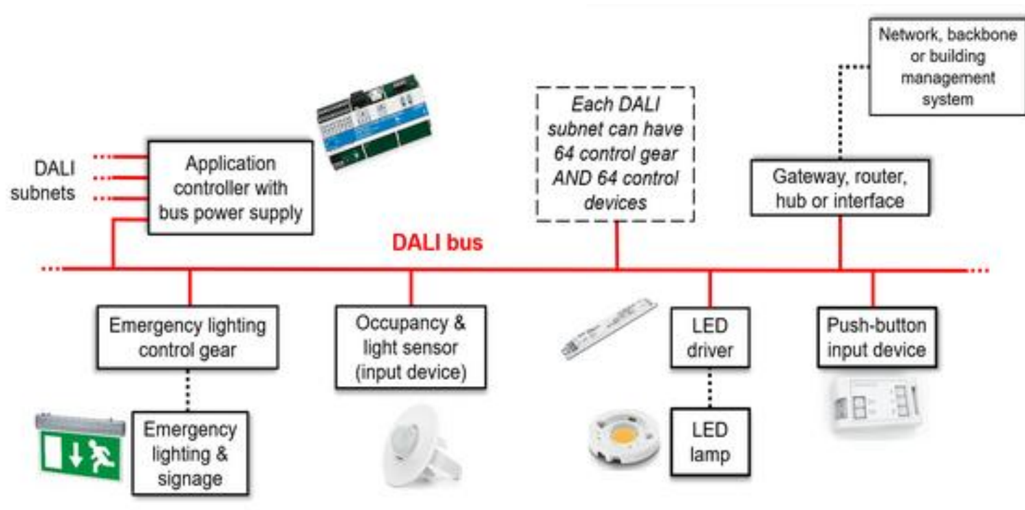
Voorbeeld van een systeem voor het beheer van de verlichting gebaseerd op DALI 2 Bron: DALI Alliance
