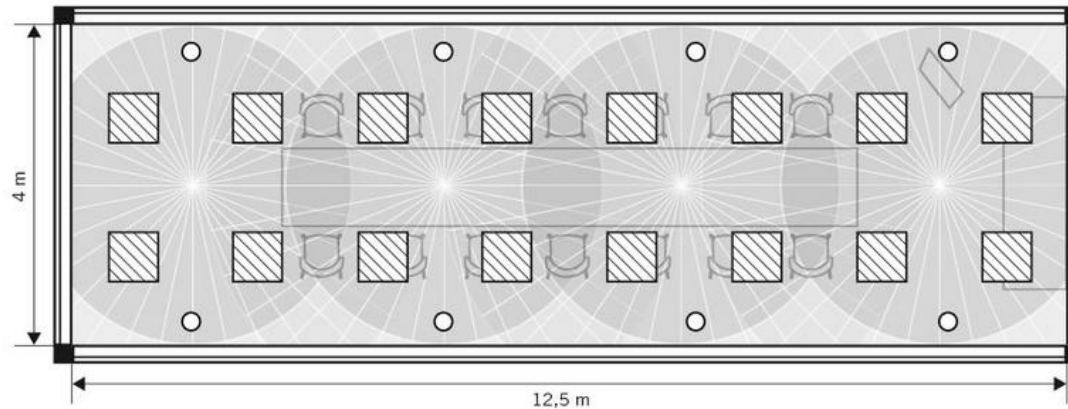
Voorbeeld van planning met automatische in- en uitschakeling door aanwezigheidsdetectie en permanente regeling van de helderheid volgens de omgevingshelderheid (geïntegreerd in de verlichtingstoestellen)
