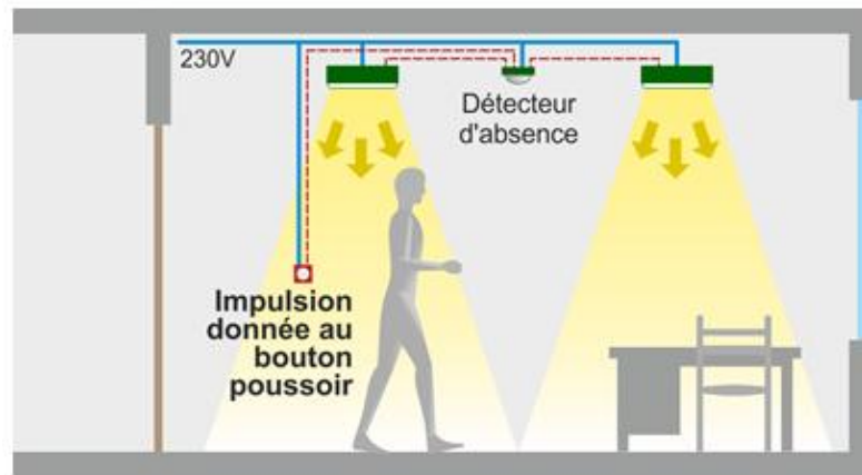
Voorbeeld van semi-automatisch beheer van de in- en uitschakeling van de verlichting in langdurig bezette lokalen
