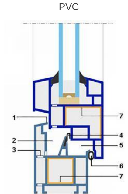
Principedoorsnede van een raamprofiel
