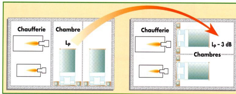
Figure 28 - Amélioration de l'isolement acoustique en réduisant la surface de contact avec la chaudière
