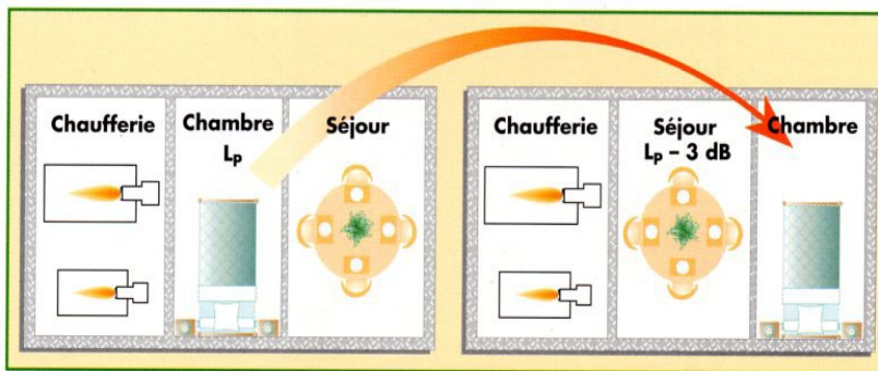
Figure 29 - Amélioration de l'isolement acoustique en augmentant la surface de la pièce mitoyenne à la chaudière
