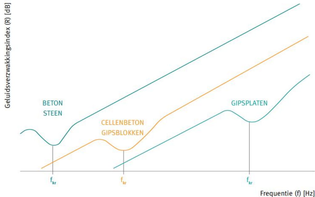
Afb. 89 Schematische evolutie van de geluidsverzwakingsindex van enkele wanden.
