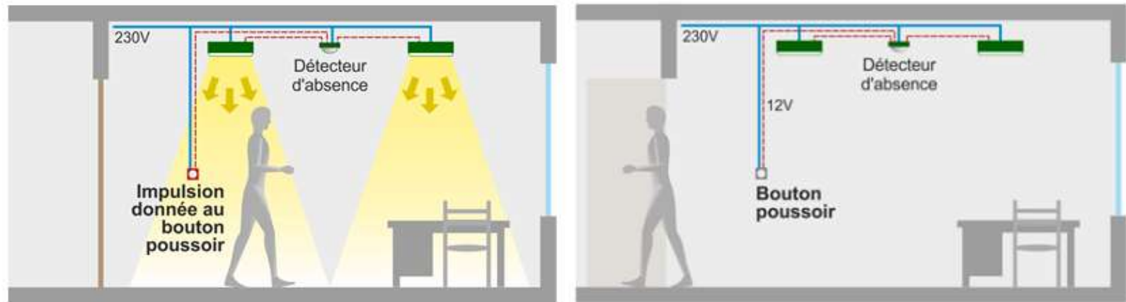
Voorbeeld van semi-automatisch beheer van de in- en uitschakeling van de verlichting in langdurig bezette lokalen
