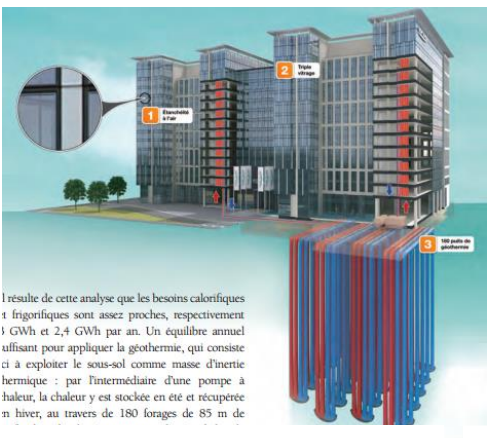
Engie Tower - Noordstation Gesloten lus 180 sondes – diepte 85 m
