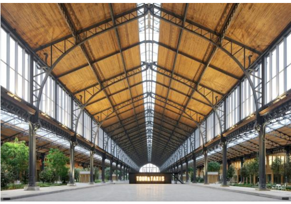
Gare Maritime - T&T Open lus 5 bronnenparen - diepte 150 m
