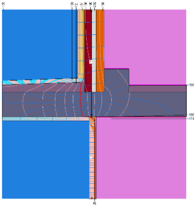
Omgeven balkon
