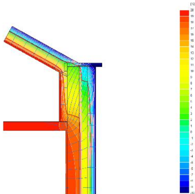
aansluiting hellend dak
