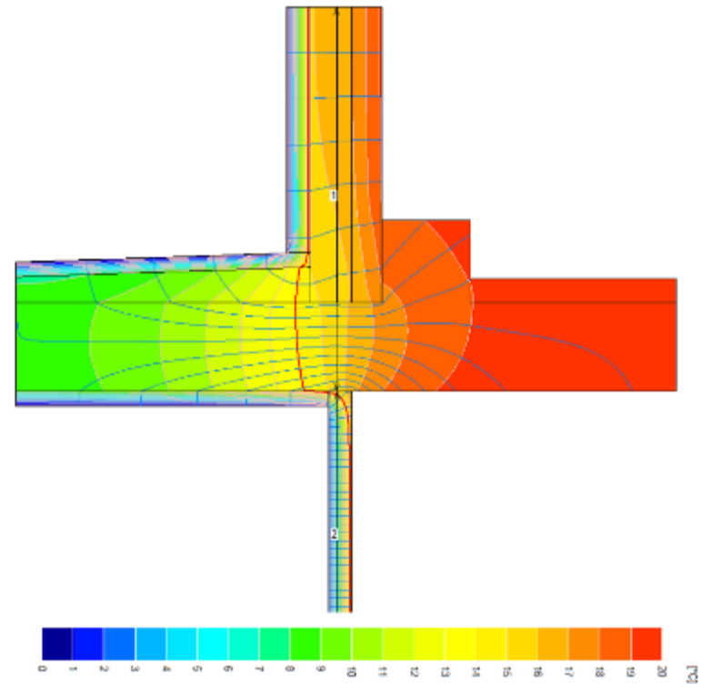
Omgeven balkon
