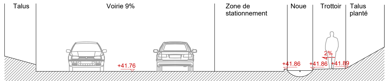
Profil 1_9% openbare weg
