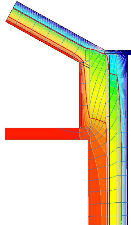
aansluiting hellend dak
