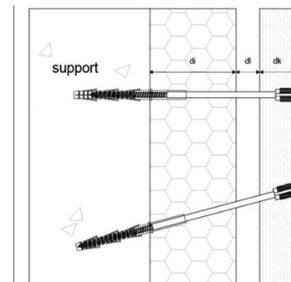
Hybride bevestiging + kleinere doorsnede = minder warmteverlies
