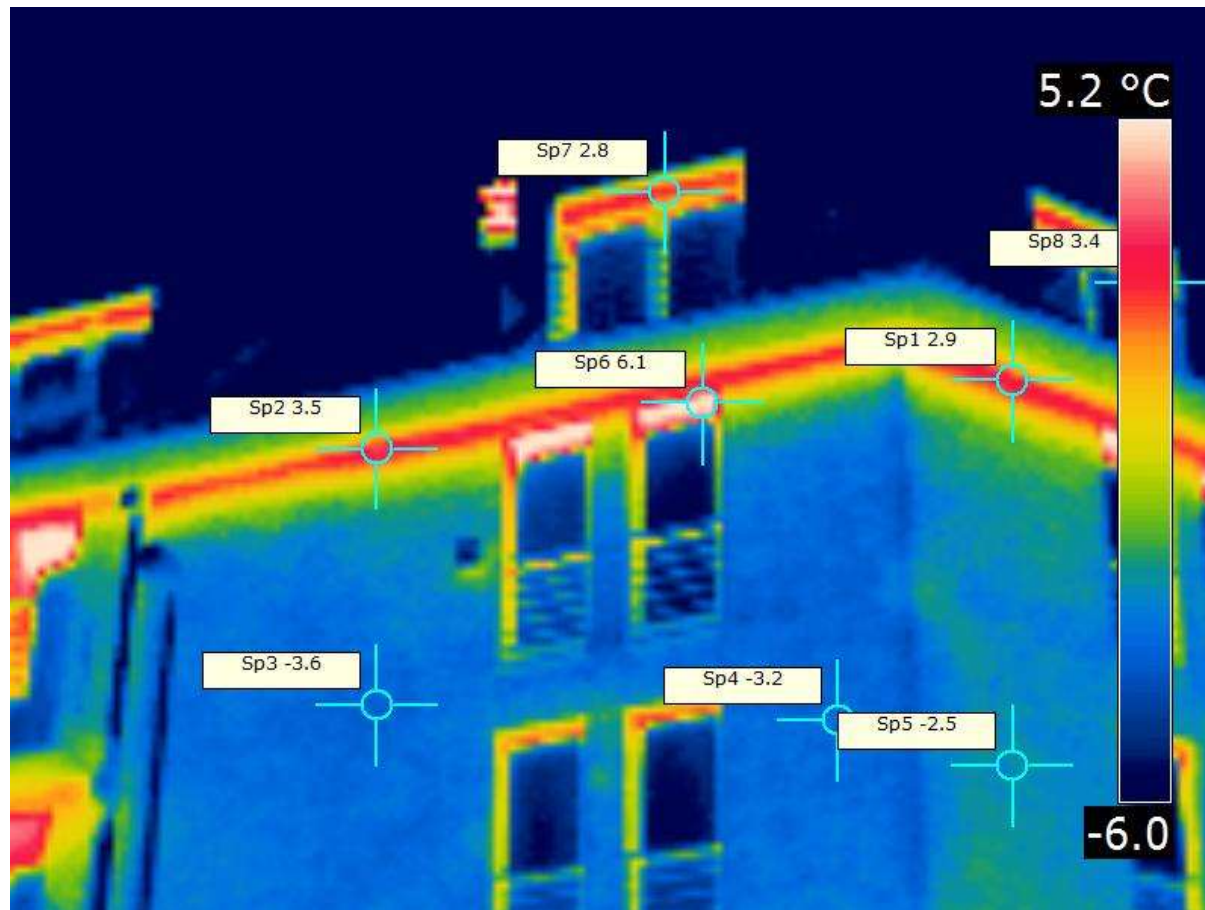
Aansluiting hellend dak
