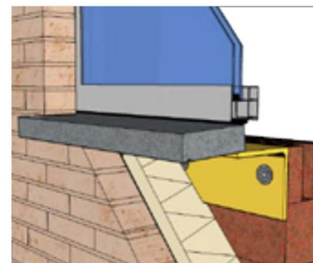
Ondersteuning arduindorpel Support seuil de pierre bleue
