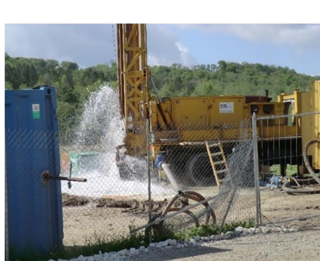
Forage du puits de production
