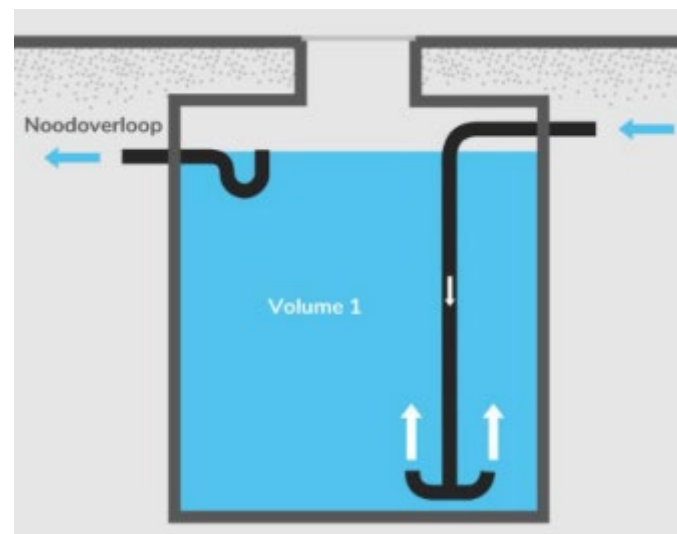
HERGEBRUIKTANK
