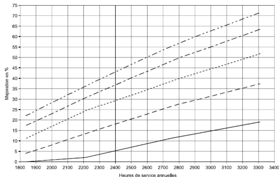
Figure 11 Majoration de longueur de sonde géothermique en fonction des heures de service et la disposition de SG avec une conductivité thermique de 2\text{ W/(m·K)} et 5\text{ m} de distance entre les sondes
