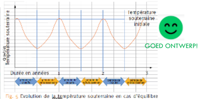
Fig. 5 Evolution de la température souterraine en cas d'équilibre thermique.
