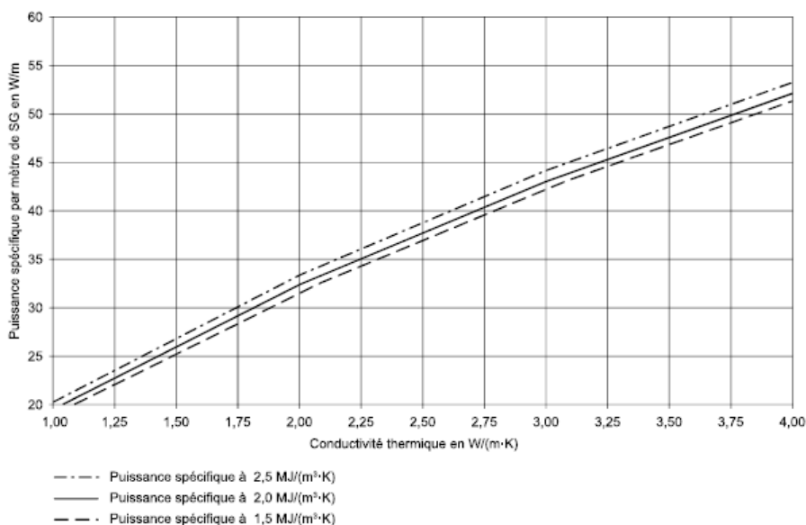
Figure 7 Puissance nominale pour 1 SG de 100 m, \varnothing 32 mm, duplex, à 10^{\circ}\text{C} de température du sol moyenne et 1850 h de pleine charge, avec différentes conductivités thermiques et capacités thermiques du terrain
