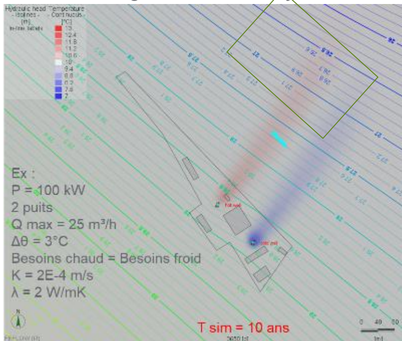
Fig. 4 Evolution de la température souterraine en cas de déséquilibre
